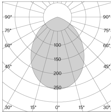
w225 Ion 3000 K weit
