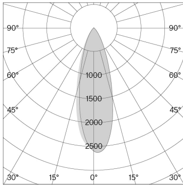
w225 Ion 3000 K schmal
